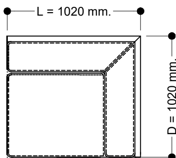
CORNER WEDGE ITEM CODE : 85018
